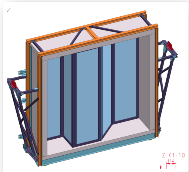
Prüfaufbau Eckverglasung
