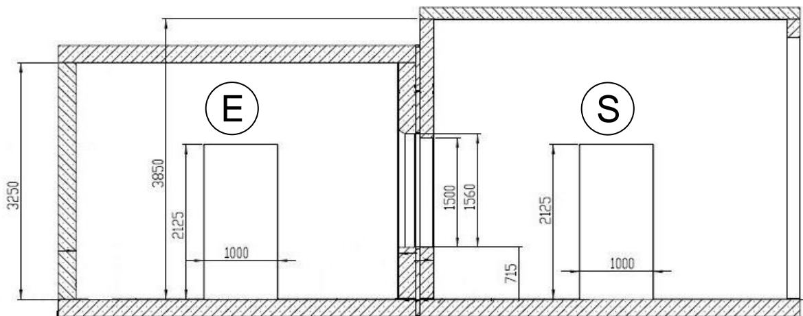
Seitenansicht Wandprüfstand
