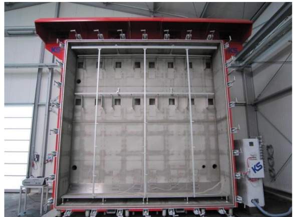
Rauchprüfkammer 5 x 5 m – Innenansicht
