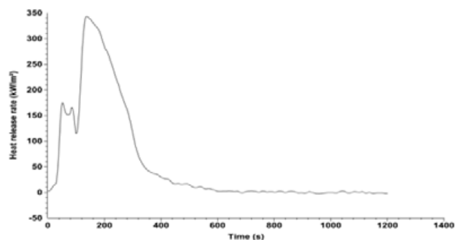
Darstellung der ermittelten Wärmefreisetzungsrate
