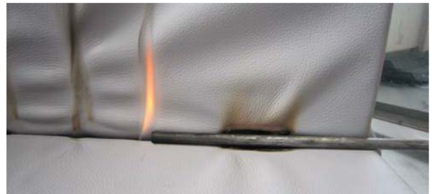
Brandversuch Gasflamme Polstermöbel
